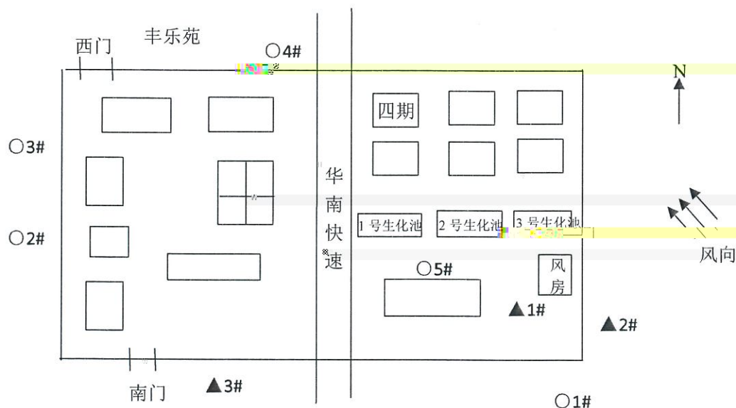
3 测点分布示意图及简要说明 (注: ▲代表噪声检测点, ○代表无组织废气检测点)
